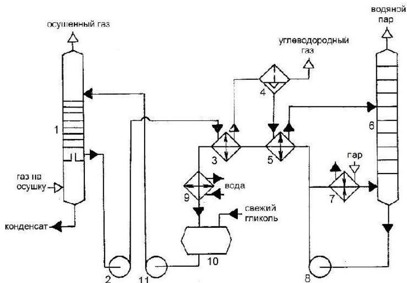
Рисунок 2.1 – Технологическая схема установки осушки газа:
