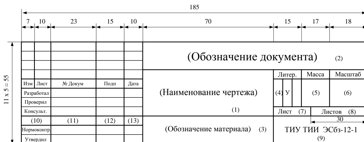
Рисунок 1 – Форма основной надписи на чертеже
