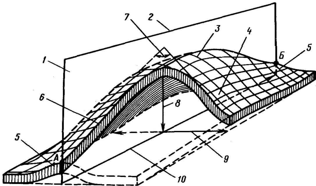
Рис. 3 – Элементы антиклинальной складки (1/4 складки условно удалена). 1 – осевая плоскость; 2 – ось; 3 – свод (замок); 4 – крыло; 5 – периклиналиль; 6 – шарнир АБ; 7 – угол; 8 – амплитуда; 9 – ширина; 10 – длина
