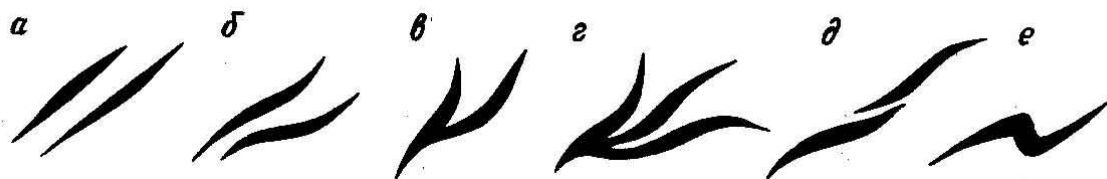
Рис. 7. Типы складок в плане: а – прямолинейные, б – дугообразно изогнутые,
