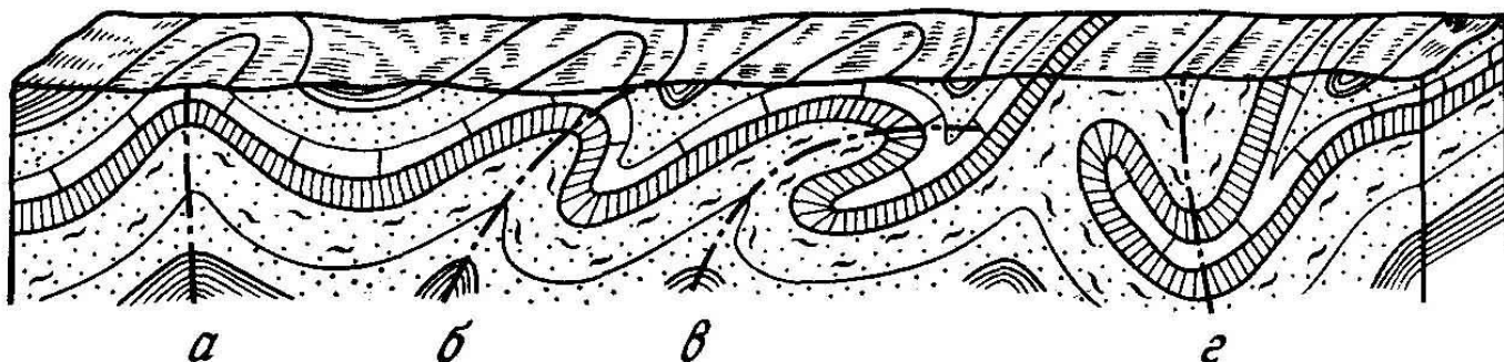
Рис. 5 - Типы складок по положению осевой поверхности:
