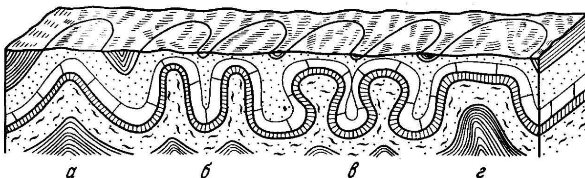
Рис. 6. Типы складок по положению крыльев:
