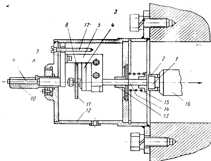
Рис. 6. Датчик осевого смещения.
