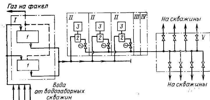
Рис. 4. Технологическая схема блочной кустовой насосной станции.
