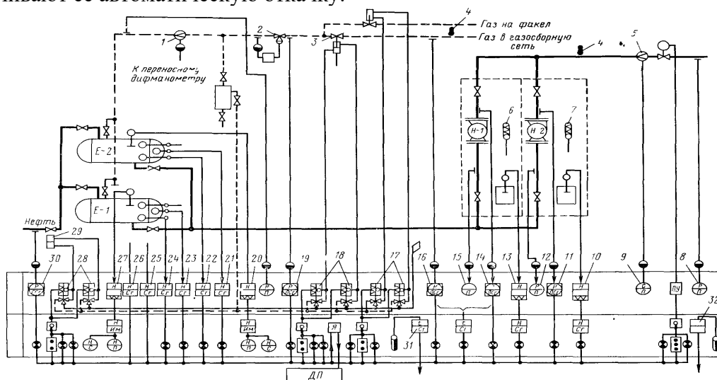
Рис. 13.Схема автоматизированной блочной дожимной насосной станции
