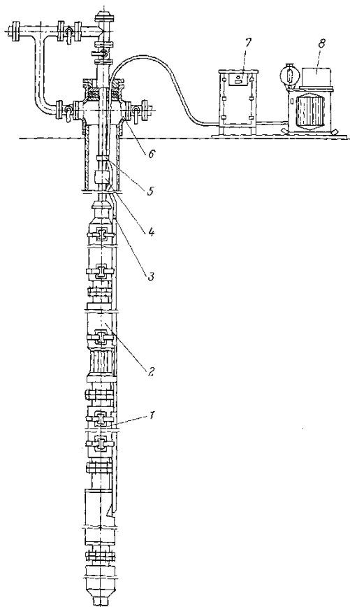
Рисунок 2.1 – Схема УЭЦН
