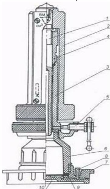
Рисунок 2 - Прибор ВМ-6
