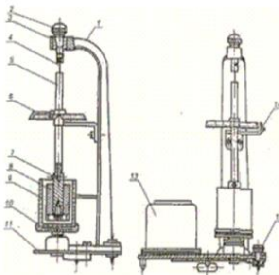
Рисунок 1 – Прибор СНС-2
