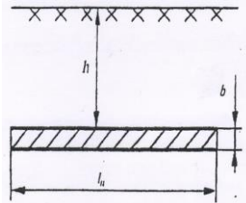
Рисунок 3. Полоса связи заземлителей
