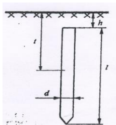
Рисунок 1 Вертикальный заземлитель
