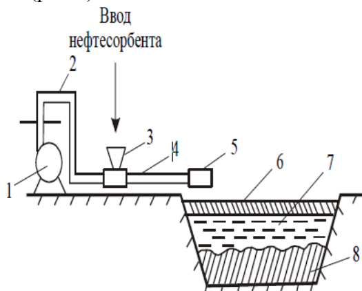
Рисунок 3 - Принципиальная технологическая схема обработки поверхности ША 1-слой плавающей нефти, 2- эмульсионный слой, 3-вода (БСВ), 4- илам, 5-компрессор, 6-ввод нефтесорбента, 7- распылитель
