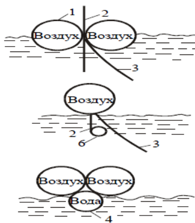
Рисунок 2 - Конструкции бонового ограждения
