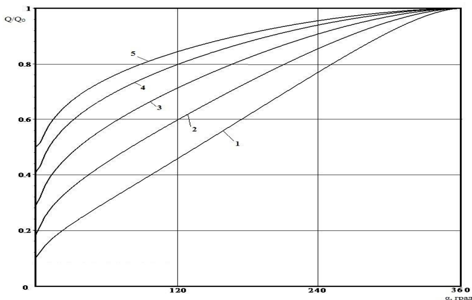
Рисунок 2 – Зависимости дебита скважины с разными углами раствора пронизываемой дуги.
