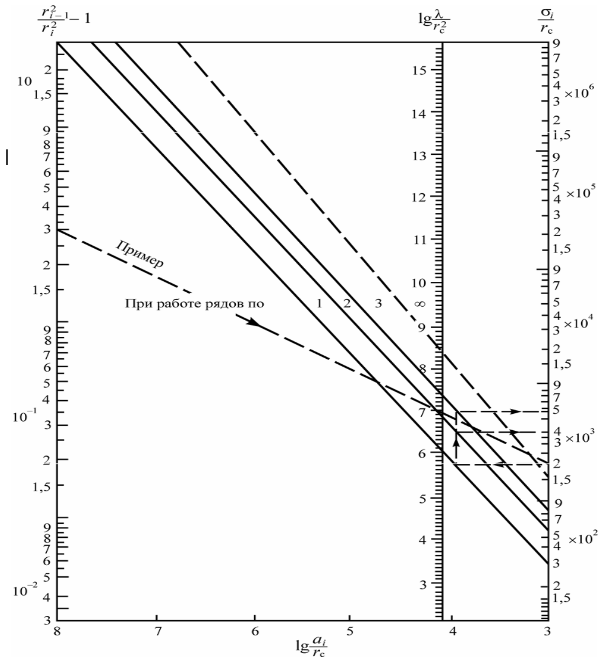
Номограмма расстояний между скважинами в рядах
