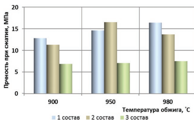
Рис. 6. Результаты испытания образцов на прочность
