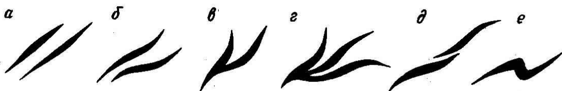
Рис. 7 - Типы складок в плане: а – прямолинейные, б – дугобразно изогнутые, в – ветвящиеся, г – виргирующие, д – кулисообразные, е – сигмовидная
