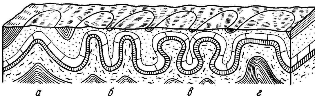
Рис. 6 - Типы складок по положению крыльев:
