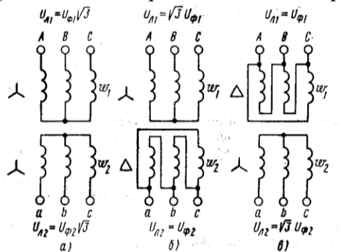
Рисунок 36. Соединения обмоток трехфазного трансформатора: соединение обмоток звездой (а); соединение первичных обмоток звездой, вторичных -треугольником (б); соединение первичных обмоток треугольником, вторичных - звездой (в).
