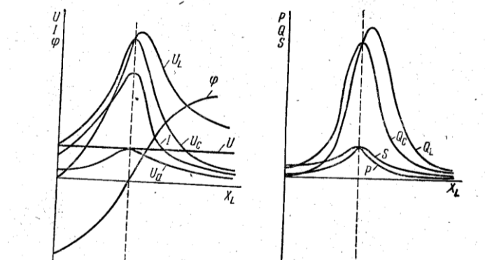
Рисунок 10. Резонансные кривые
