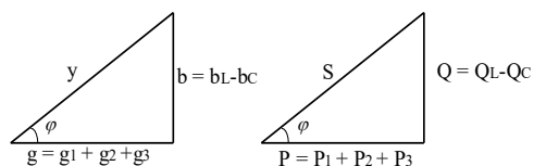
Рисунок 27. Треугольники проводимостей и мощностей
