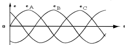
Рисунок 12. Графики мгновенных ЭДС фаз A, B, C генератора (начальная фаза \varphi_A=0^\circ )
