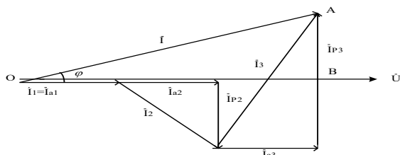
Рисунок 26. Векторная диаграмма напряжений и токов
