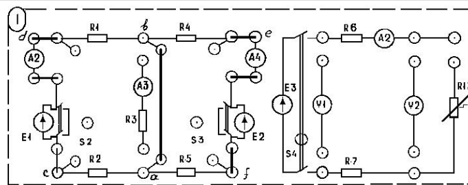
Рисунок 7. Опыт короткого замыкания
