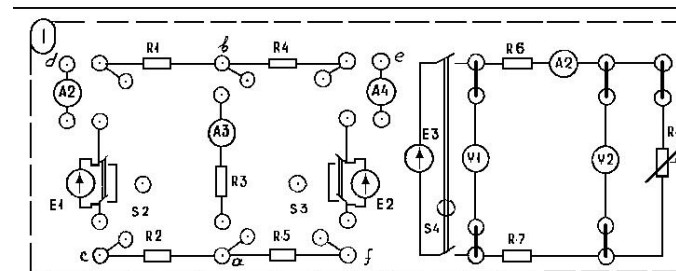
Рисунок 8. Схема цепи
