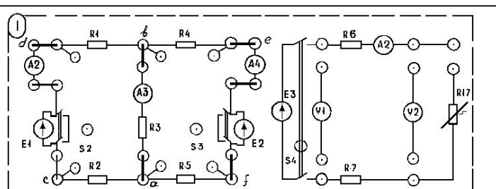
Рисунок 5. Схема цепи.
