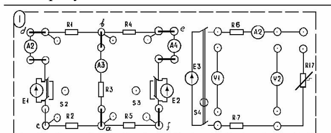
Рисунок 2. Схема цепи
