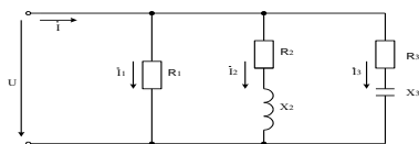
Рисунок 25. Параллельное включение приемников синусоидального тока
