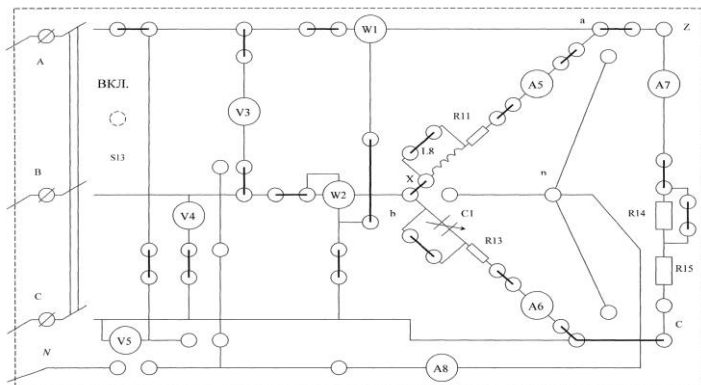
Рисунок 23. Схема установки
