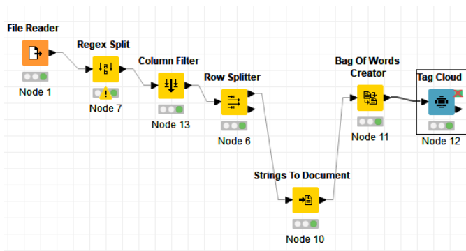
Пример схемы процесса в KNIME Analytics Platform
