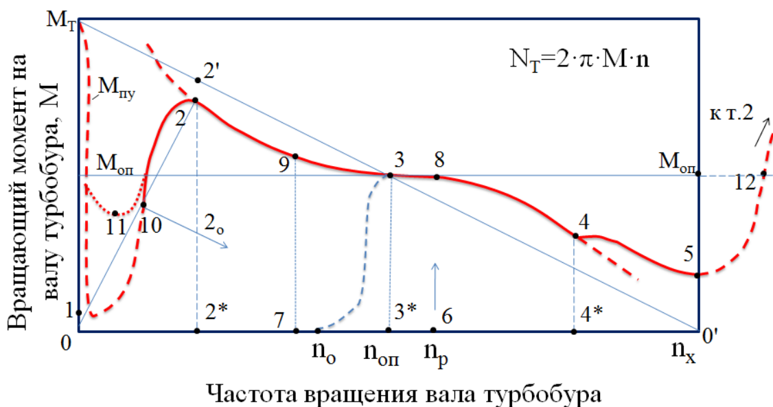
Рисунок 3.1 - Характеристика турбобура
