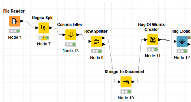
Пример схемы процесса в KNIME Analytics Platform
