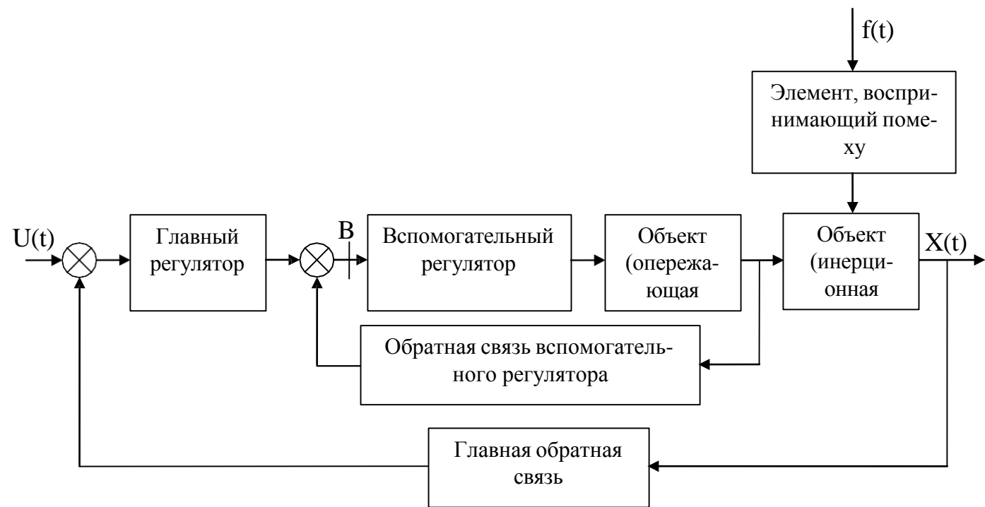
Рисунок 1. Структурная схема системы каскадного регулирования
